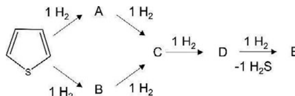
Rysunek 1. Proces hydroodsiarczania tiofenu.
