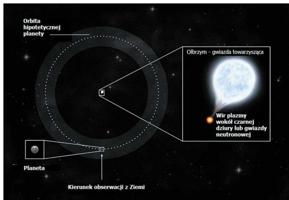
▲ Schemat układu M51-ULS-1, w którym znajduje się planeta
