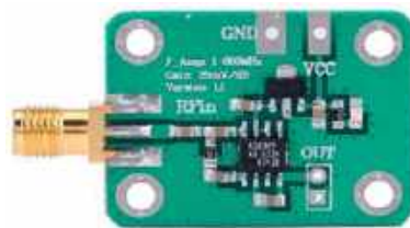
Rys. 2. Płytki prototypowa układu AD8307
