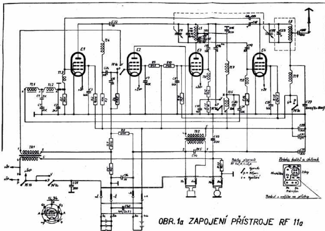
Rys. 1. Schemat ideowy radiostacji RF-11a
