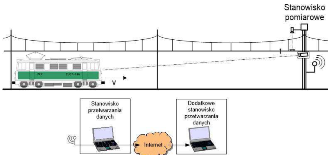
Rysunek prezentuje działanie nowoczesnego systemu do wykrywania usterek pantografów
