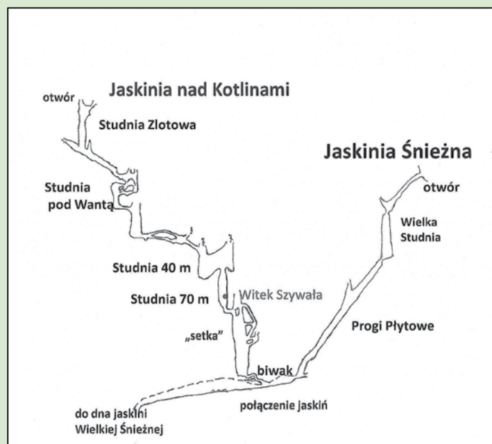
Rok 1970. Przekrój górnej partii Jaskini Wielkiej Śnieżnej.
