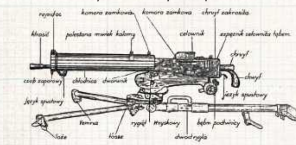
Ryc. 131. Ciężki karabin maszynowy wz. 30.
