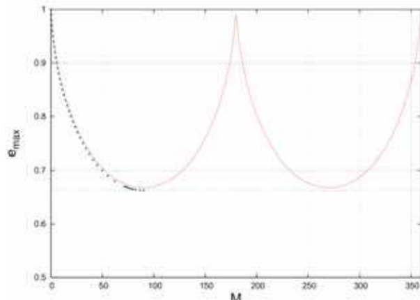
Rys. 3. Promień zbieżności szeregu Lagrange'a w funkcji anomalii średniej. Linia czerwona zaznaczona jest maksymalna wartość mimośrodu, dla którego rozważany szereg jest zbieżny, linia zielona to teoretycznie wyznaczona granica Laplace'a, punkty niebieskie to promień zbieżności policzony teoretycznie.
