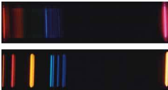
Fot. 3. Nawet tanie okulary dyfrakcyjne pozwalają na analizę kolorów w wyladowaniu elektrycznym (w tzw. rurkach Plückera). Plazma wodorowa (również ta na obrzeżach w reaktorze termojądrowym) jest różowa, plazma helowa – pomarańczowa. W rzeczywistości, jest to wiele linii (w wodorze, nie do końca dysocjowanym, oprócz 4 linii Balmera widać również pasma H 2 ).
