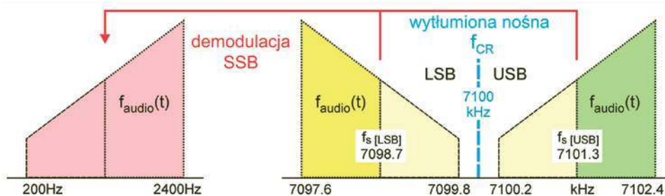
Rys. 7. Demodulacja SSB przy odbiorze w paśmie 40 m
