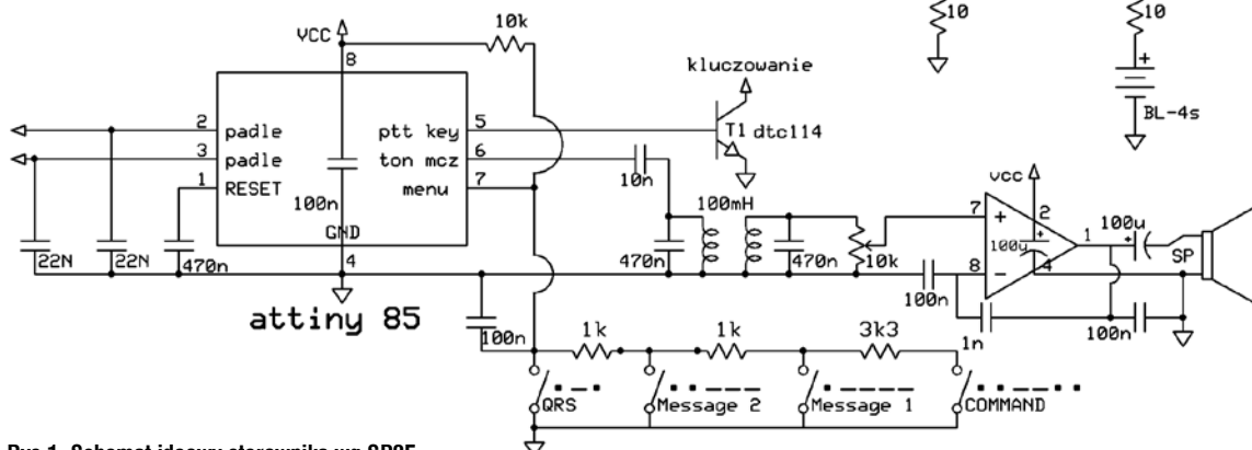
Rys 1. Schemat ideowy sterownika wg SP2FP
