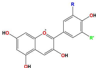
Rys. 10. Budowa cząsteczek cyjanidyny, delfinidyny, pelargonidyny.
