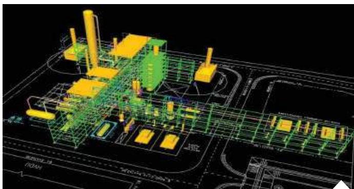
Wstępny model 3D instalacji Hydrokrakingowego Bloku Olejowego | fot. mat. pras.
