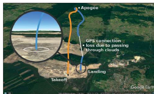
Tor lotu rakiety i CanSata, który stworzyli uczniowie raciborskiego „Mechanika” na podstawie danych z modułu GPS oraz wysokości obliczonej ze wzoru barometrycznego
