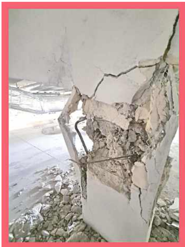
Tak wygląda uszkodzony słup żelbetonowy podpierający nieckę basenową
