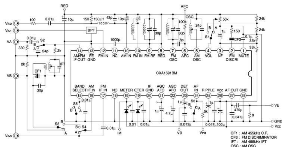
Rys. 1. Schemat ideowy odbiornika z wykorzystaniem układu CXA1691BM
