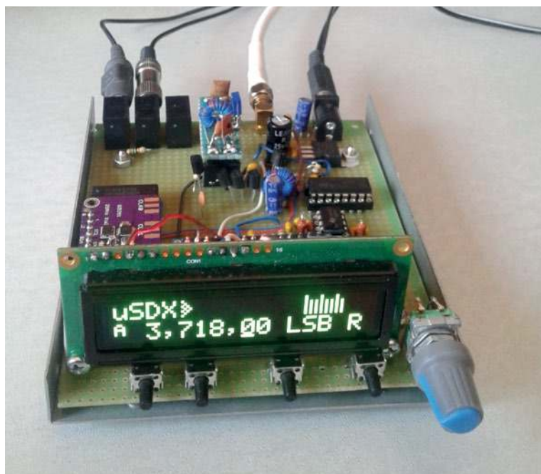
Eksperymentalny transceiver μSDX konstrukcji SP5GNI
