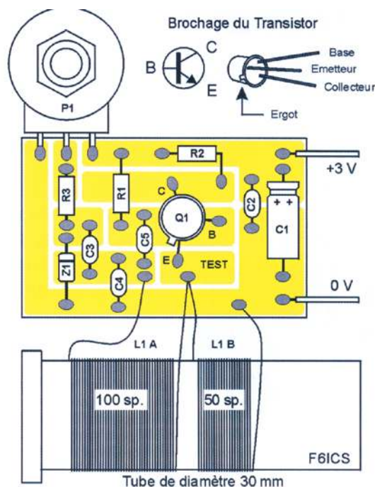
Rys 2. Schemat ideowy generatora BFO wg F6ICS
