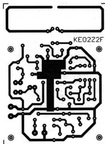
Rys. 2 Szkic PCB wskaźnika
