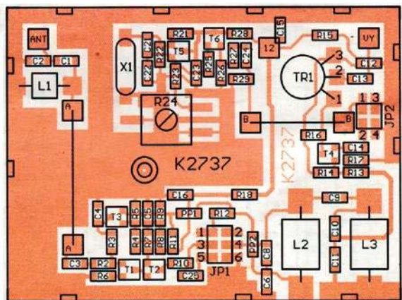
Rys. 5. Płytki drukowane i rozmieszczenie elementów na PCB konwertera
