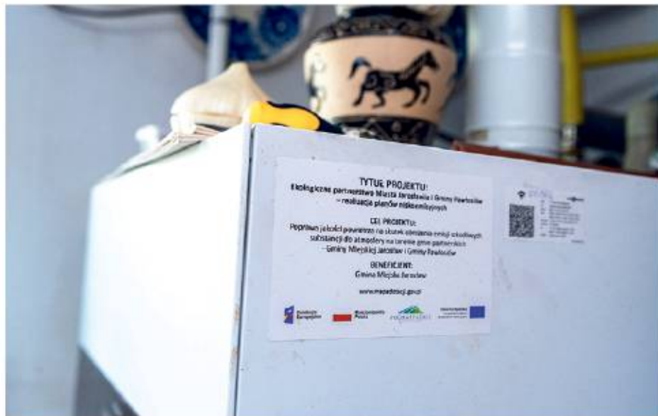
Instalacja kotłów gazowych kondensacyjnych oraz kotłów na biomase.
