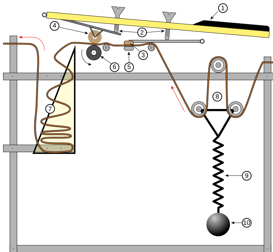
Rysunek 3. Schemat mechanizmu Mellotronu. Naciśnięcie klawisza (1) powoduje, że dwie śruby (2) łączą płytkę dociskową (3) z głowicą taśmy (5) oraz koło dociskowe (4) z obracającym się w sposób ciągły wałkiem napędowym (6). Taśma jest naciągana ze stałą prędkością, równoważona sprężyną naciągową (8...10) i tymczasowo przechowywana w pojemniku (7) do momentu zwolnienia klawisza
