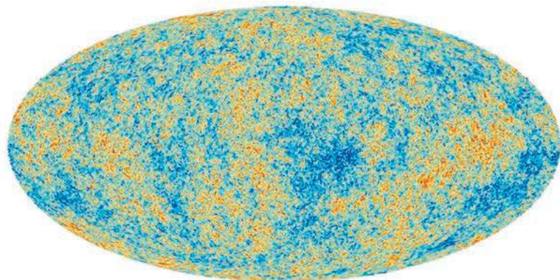
Mapa mikrofalowego promieniowania tła. Różnice w kolorach odpowiadają różnicom temperatur
