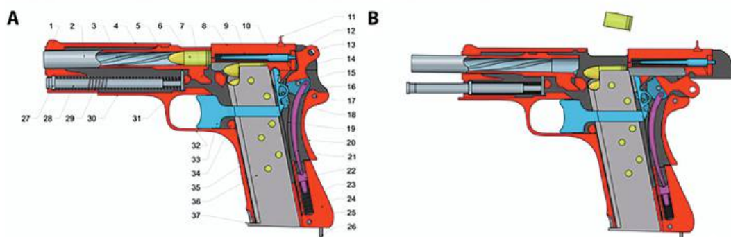
Budowa pistoletu Vis | fot. arch./d
