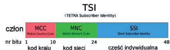
Rys. 1. Struktura identyfikatora stacji w systemie TETRA
