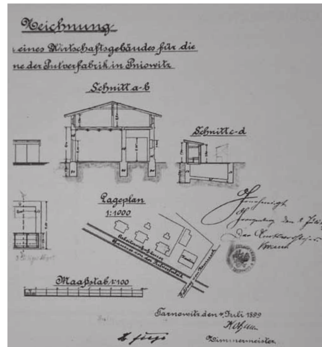
Wykonany w 1899 r. projekt budynku gospodarczego przy dawnej kantine przy obecnej ul. Obrońców Pokoju w Boruszowicach
