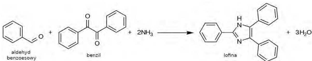
Rys. 4 – Schemat reakcji syntezy lofiny
