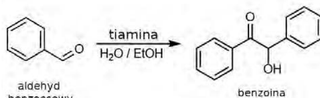
Rys. 2 – Schemat reakcji syntezy benzoiny
