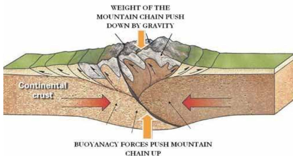
Ilustracja ukazująca balans sił w skorupie ziemskiej. Ten balans czterech sił zależy od wzrostu, pograżania się gór czy ich fałdowania.
