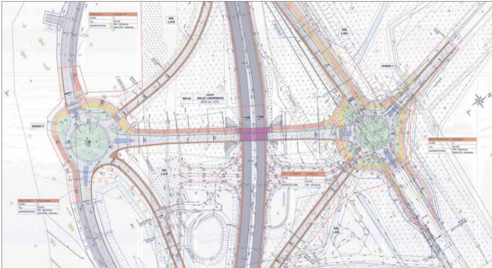
Projekt przedstawia węzeł Orłąt Lwowskich. Przez środek na szaro zaznaczono przebieg DK79. Po prawej stronie rondo od strony Dąbrowy Narodowej, a po lewej rondo, które między innymi rozprowadzi ruch na teren JOG-u. Oba rondo połączy wiadukt nad DK 79
