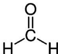
Rys. 1 – Wzór strukturalny aldehydu mrówkowego
