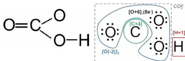
Rys. 2. Anion wodorowęglanowy – wzór strukturalny oraz schemat graficzny otoczenia poszczególnych rdzeni. Zapis wg oryginalnej notacji prof. Górskiego: {}^{\delta}HCO_3^{-} . Poniżej – etapy opisu anionu HCO_3^{-} w notacji macierzowej:
