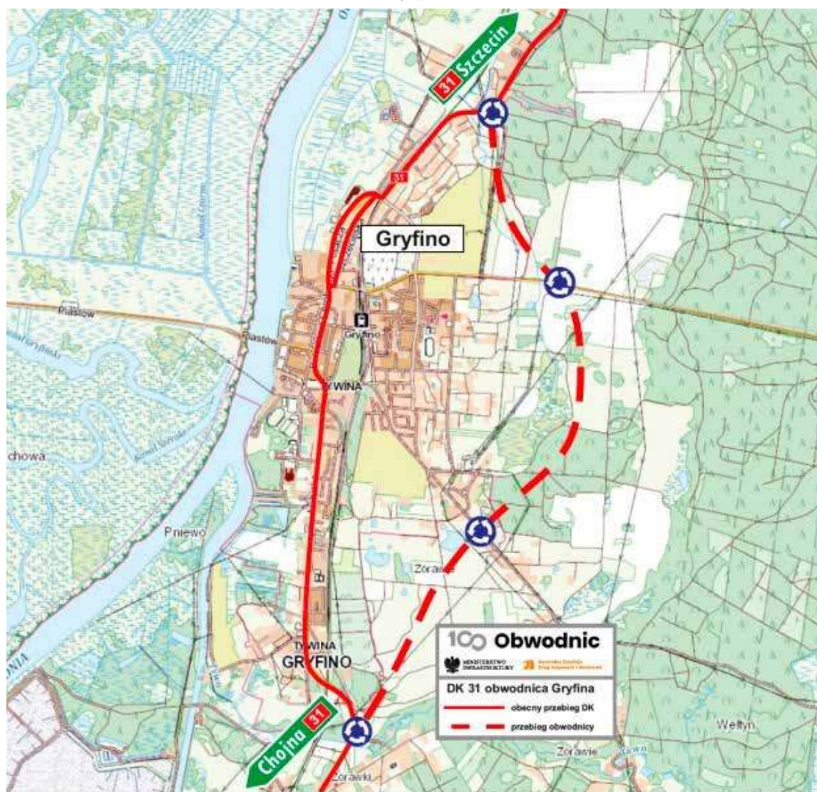
Plan obwodnicy Gryfina
