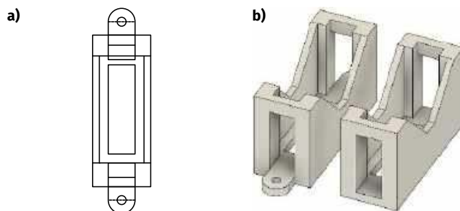
Rysunek 8. Element do montażu przełączników: szkic (a), dwa warianty stworzone z tego szkicu (b)
