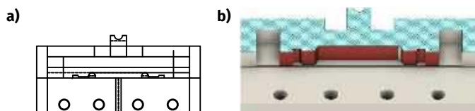
Rysunek 3. Przetątnik trzypozycyjny: szkic (a) i przekrój modelu (b)
