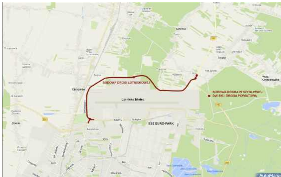
Plan drogi lotniskowej i ronda w Szydłowcu.
