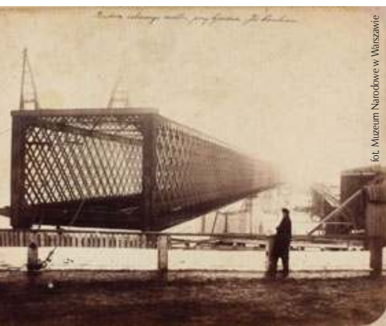
Montaż konstrukcji żelaznej przęsła mostu Kierbedzia na Wiśle, Zakład Fotograficzny Karola Beyera w Warszawie, 1864
