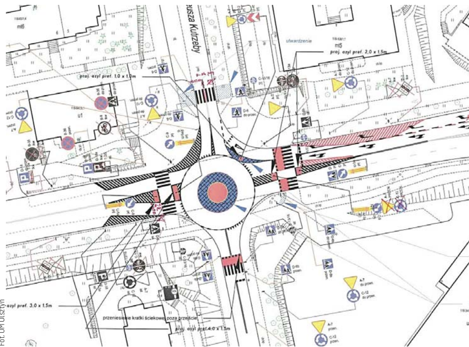
Schemat nowej organizacji w okolicach ronda Wilczyńskiego/Kutrzeby/Barcza
