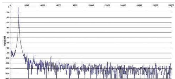
Rys. 2. Zniekształcenia harmoniczne
