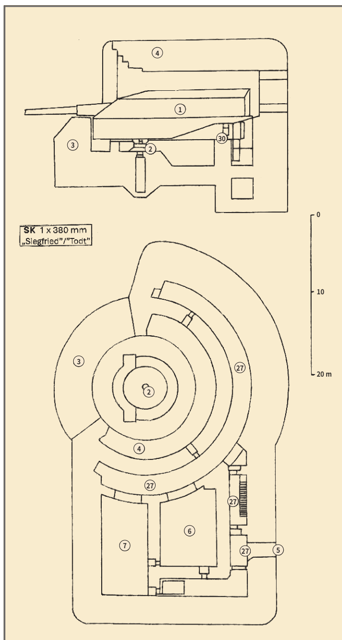
Schron-stanowisko bojowe typu SK (baterie Siegfried / Todt ). Opis oznaczeń na końcu artykułu.
