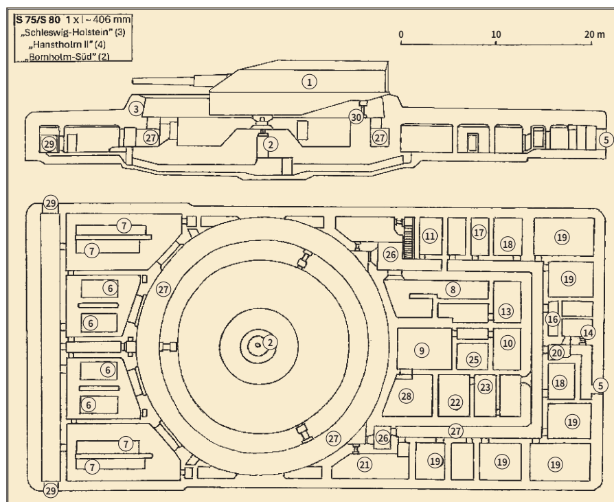
Schron-stanowisko bojowe typu S 75/80 ( Schleswig-Holstein, Bornholm-Süd, Hansthalm II ). Opis oznaczeń na końcu artykułu.
