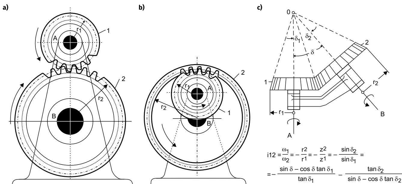
Rysunek 2. Przekładnie zębate: przekładnia prosta (a) i przekładnia z wewnętrzną zębatką (b). Linia przerywaną zaznaczono średnice podziałowe kół zębatych r1 i r2, ich styczna wyznacza idealny dystans między kołami zębatymi, a stosunek – przełożenie przekładni, którą określa też liczba zębów. Średnice podziałowe koła zębatego zależą od geometrii zębów. Przekładnia stożkowa i sposób wyznaczania kątów stożków (c)
