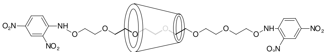
rotaksan z cyklodekstryną
