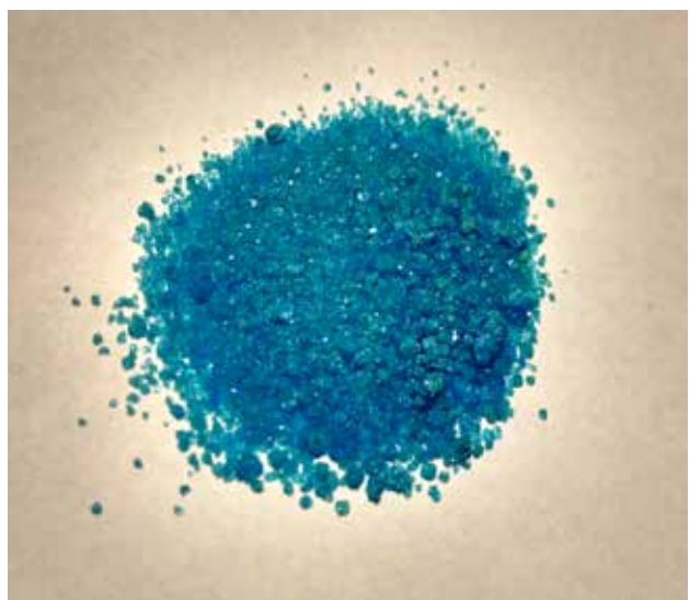
Fot. 3 – Kryształy uwodnionego siarczynu(VI) miedzi(II)
