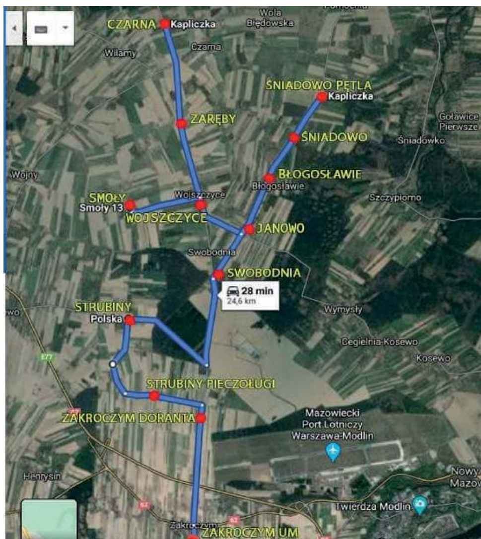
Trasa linii Zakroczym - Śniadowo Pętla
