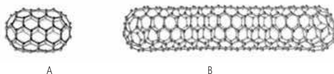
Rys. 16. (A) Struktura cząsteczki fullerenu C_{540} , (B) nanorurka z zamkniętymi końcami.
