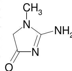
Rysunek 9. Wzór cząsteczki kreatyny
