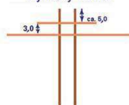
Rys. 19. Wymiary anteny planarnej na pasmo 13 cm. Elementy są wykonane z blachy mosiężnej lub miedzianej o grubości 1 mm, a falowód środkowy z rurki miedzianej o średnicy zewnętrznej 22 mm i wewnętrznej 20 mm. Do punktu zasilania podłączony jest kontakt środkowy gniazdka koncentrycznego. Należy stosować gniazdka dobrej jakości z kołnierzem montażowym i izolatorem teflonowym
