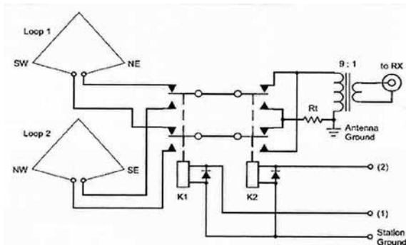
Rys. 4. Schemat przełącznika przekątnikowego
