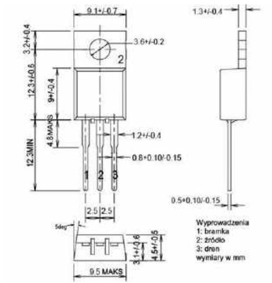
Rys. 3. Obudowa RD16HHF1
