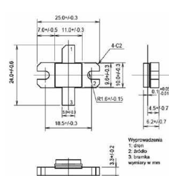
Rys. 5. Obudowa RD100HHF1
