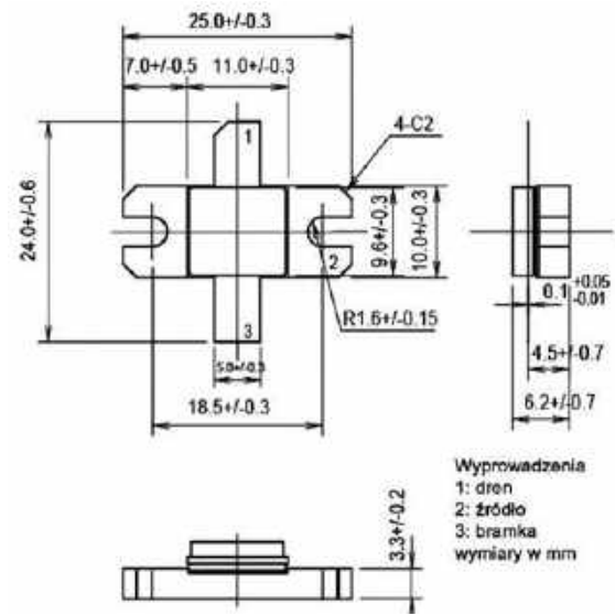
Rys. 4. Obudowa RD70HHF1
