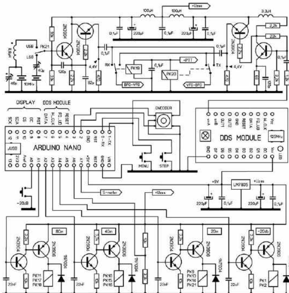
Rys. 5. Schemat układu sterowania Arduino Nano z modułem DDS
