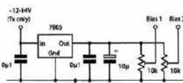
Rys. 2. Schemat układu polaryzacji bramek
