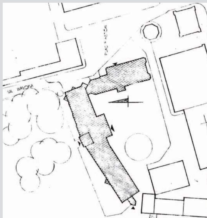
Rzut z góry na planowany do odbudowy zamek - po prawej kościół pw. Św. Apostołów Piotra i Pawła, u góry wieża ciśnień
