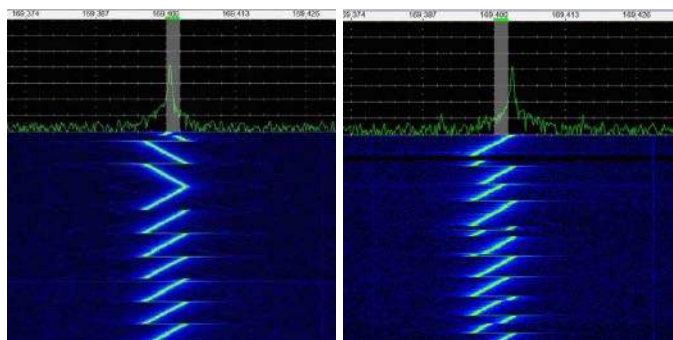
Rysunek 3. Zarejestrowany spektrogram sygnału w modulacji LoRa. Z lewej strony pokazana została tzw. preambula, niezawierająca danych, na której widać w jaki sposób wygląda sygnał modujący, którego zakres częstotliwości definiuje szerokość pasma. Zmodulowany sygnał został pokazany na przebiegu po prawej stronie
