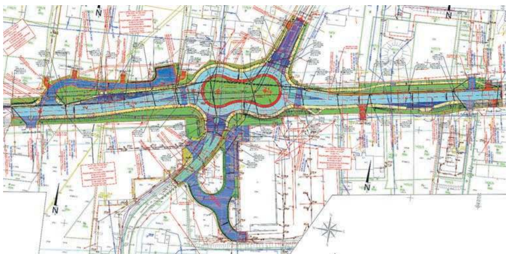
Plan sytuacyjny ronda okularowego na Mickiewicza w Alwerni. MATERIAŁ ZDW KRAKÓW
