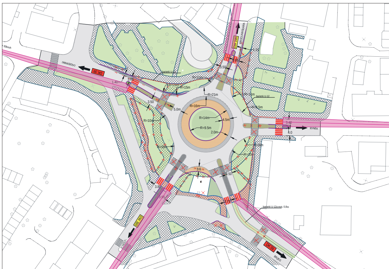
Tak wygląda techniczny plan przebudowy ronda. Zaznaczone na nim są obecne przejścia, które będą zlikwidowane oraz nowe, które mają być wybudowane
