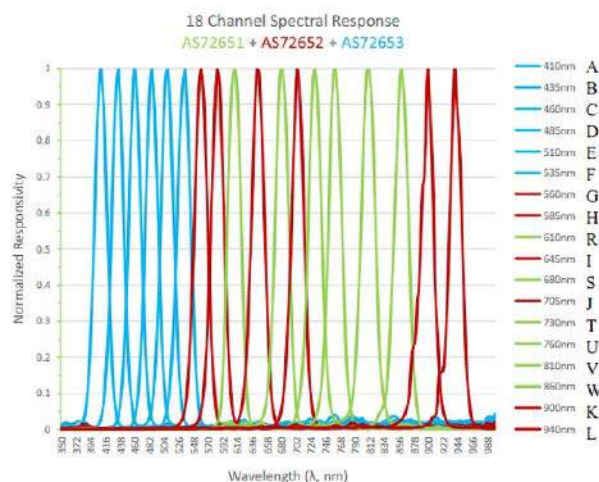
Rysunek 17. Wykres pokazujący nałożone na siebie charakterystyki spektralne czujników z serii AS7265x ( https://bit.ly/46f9c9G )
