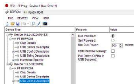
Rysunek 4. Konfiguracja prądu portu USB w programie FT Prog
