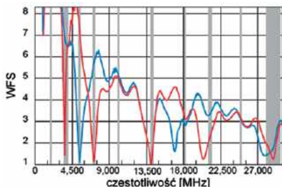
Rys. 3. WFS zmierzony dla anteny rozwieszonej na wysokości 6 m nad powierzchnią ziemi. Wykres czerwony – antena w konfiguracji dla pasm 80, 40, 20, 15, 10 i 6 m, niebieski – dla pasm 60, 20 i 10 m. Szare pionowe prostokąty obrazują położenie pasm amatorskich
