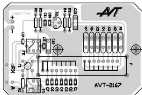
Rys. 5. Płytką drukowaną konwertera z rozmieszczeniem elementów
