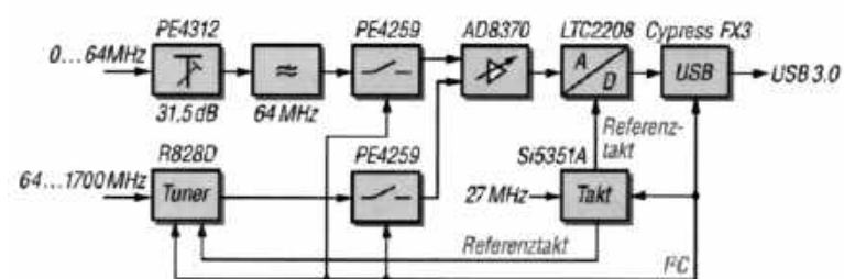
Rys. 1. Schemat blokowy odbiornika SDR RX-888 MKII
