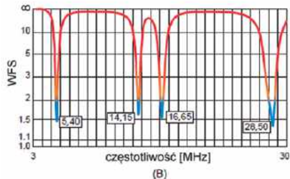
Rys. 2. Przebieg obliczony przez EZNEC: A – dla konfiguracji 80, 40, 20, 15, 10 i 6 m, B – dla konfiguracji 60 m, pracuje także w pasmach 20 i 10 m
