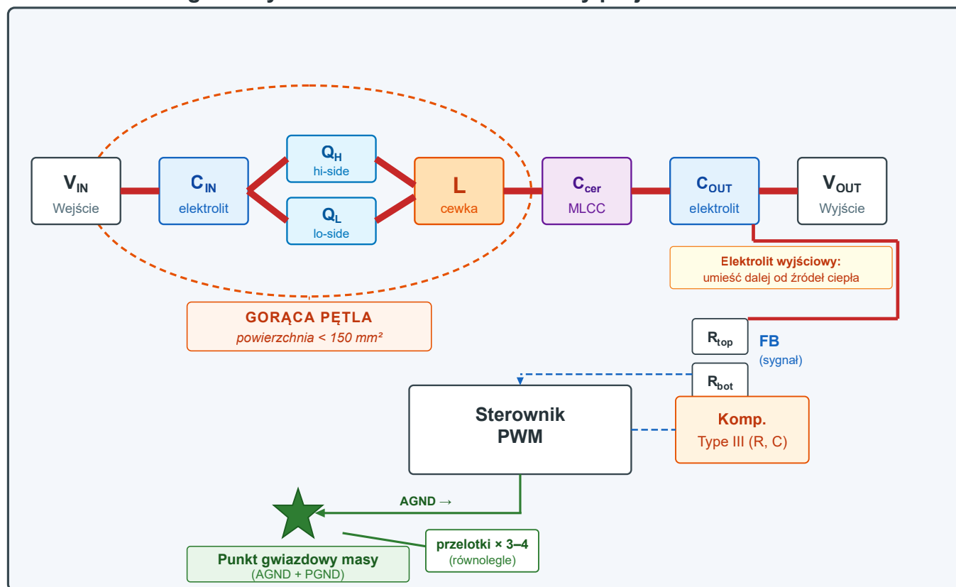
Diagram layoutu PCB – kluczowe obszary projektowania SMPS
