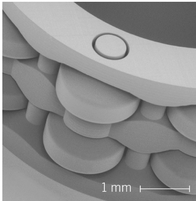
W pełni funkcjonalne, wydrukowane w 3D łożysko waleczkowe, wydrukowane w systemie druku NanoOne © UpNano GmbH
