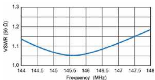
Rys. 12. Charakterystyka SWR anteny w paśmie 2 m
