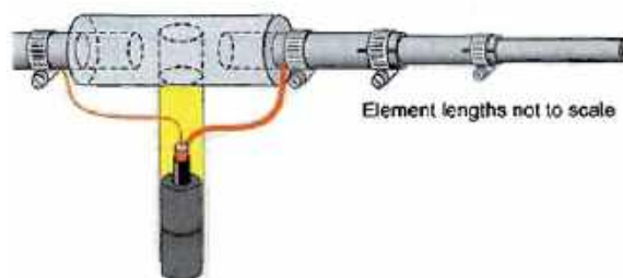
Rys. 5. Szkic montażu i podłączenia dipola
