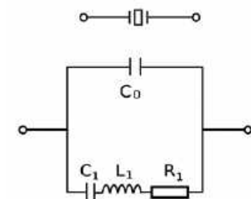
Rys. 2. Schemat zastępczy rezonatora kwarcowego
