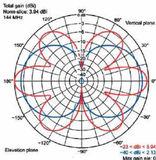
Rys. 4. Charakterystyka promieniowania, linia niebieska dla fal metrowych, czerwona dla fal decymetrowych
