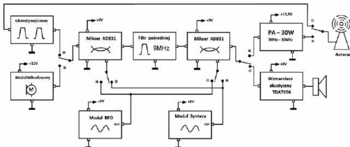
Rys. 1. Schemat blokowy rozmieszczenia i podłączenia modułów funkcjonalnych TRX-a. Przekątniki przetaczające są w położeniu do odbioru
