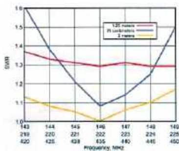
Rys. 6. Przebieg SWR w trzech pasmach amatorskich, zoptymalizowany dla 2 m FM
