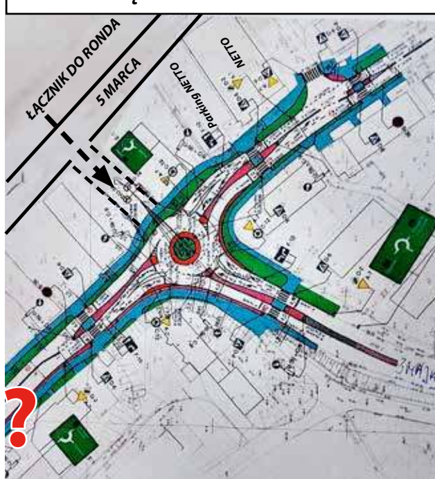
SZKIC POŁĄCZENIA 5 MARCA Z RONDEM
