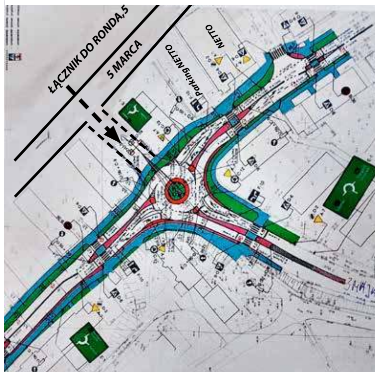
Szkic połączenia ul. 5 Marca z rondem
