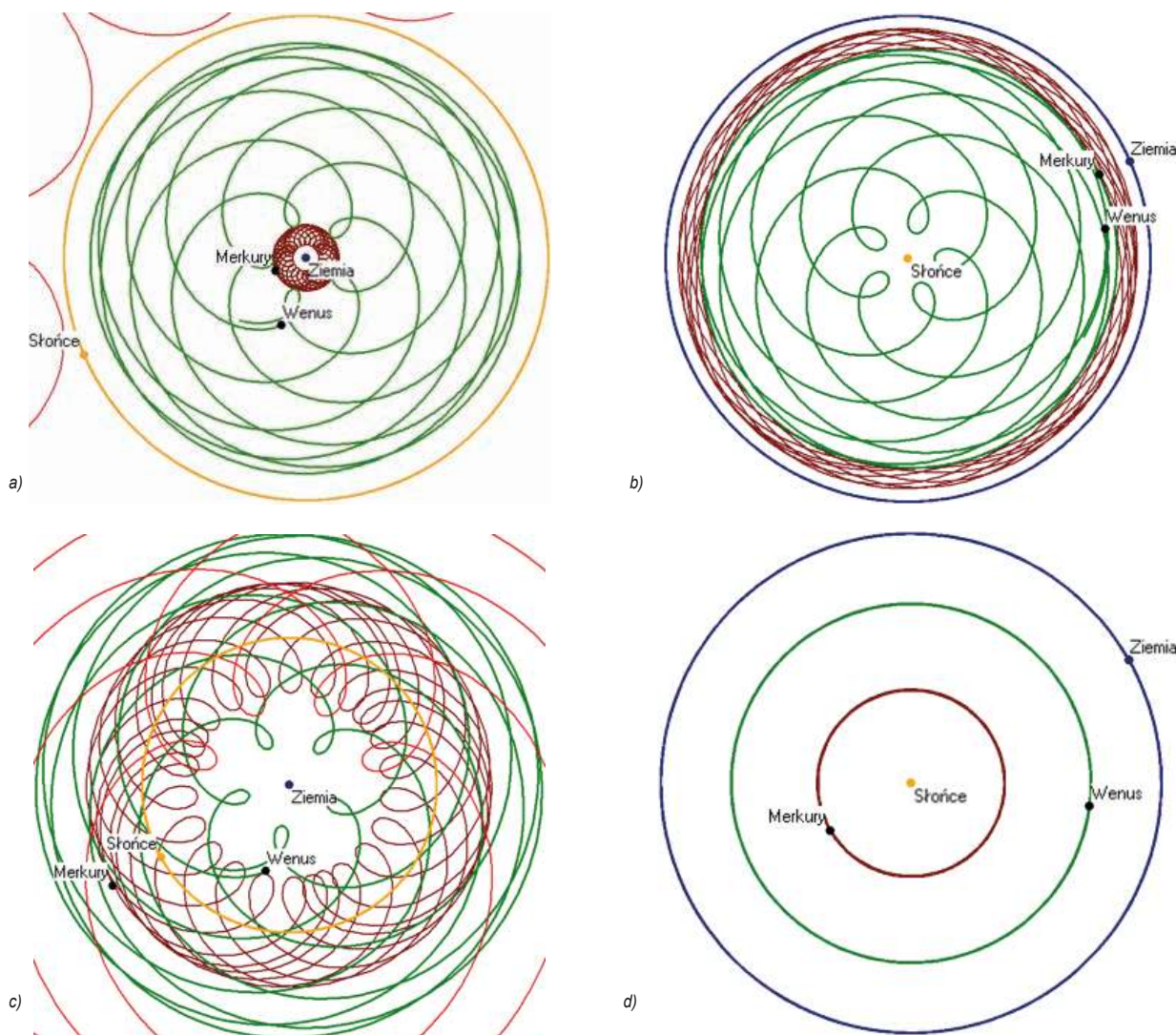
Rysunek 4. Tor planet wewnętrznych (i Słońca lub Ziemi) zakreślone w ciągu około 8 lat. Górne rysunki pokazują tor według systemu Ptolemeusza w układzie związanym z Ziemią (a) i w układzie związanym ze Słońcem (b). Dolne rysunki pokazują tor według systemu Kopernika w układzie związanym z Ziemią (c) i ze Słońcem (d). Kawałki czerwonych linii na rysunkach (a) i (c) są fragmentami toru Marsa.
