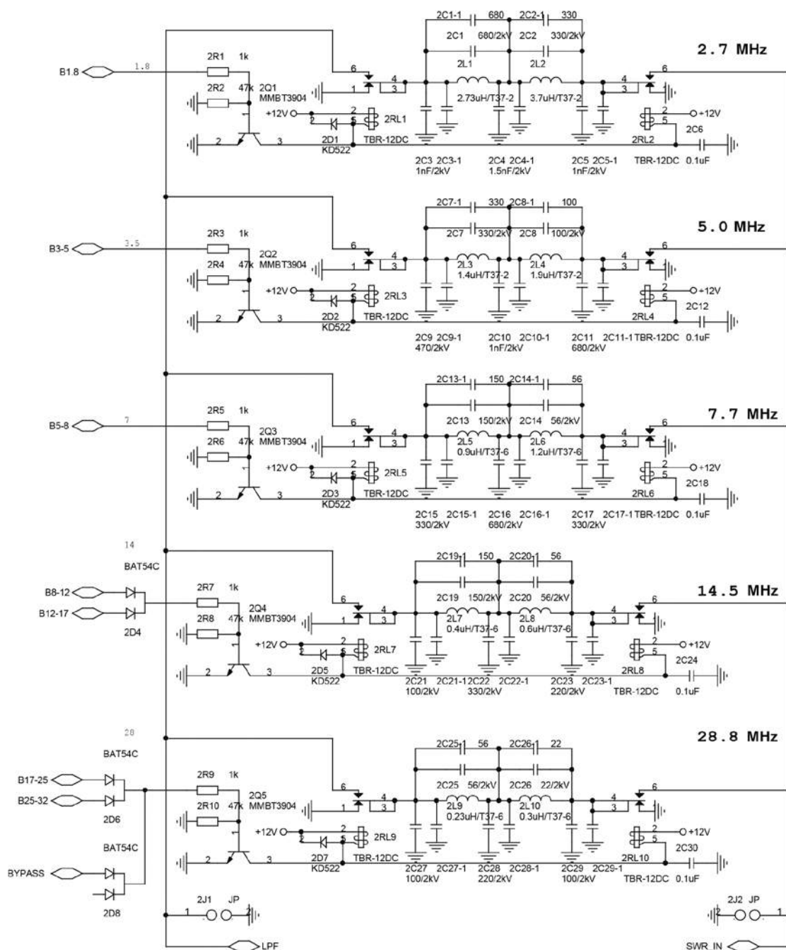
Rys. 11. Schemat ideowy filtrów dolnoprzepustowych
