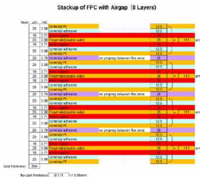
Rysunek 5. Budowa stosu 8-warstwowego obwodu elastycznego ze szczelina powietrzna
