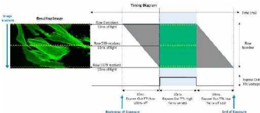
Rysunek 20. Zastosowanie metody określanej mianem pseudo-global shutter do rejestracji obrazu w warunkach synchronizowanego oświetlenia preparatu mikroskopowego ( http://t.ly/qTEn1 )
