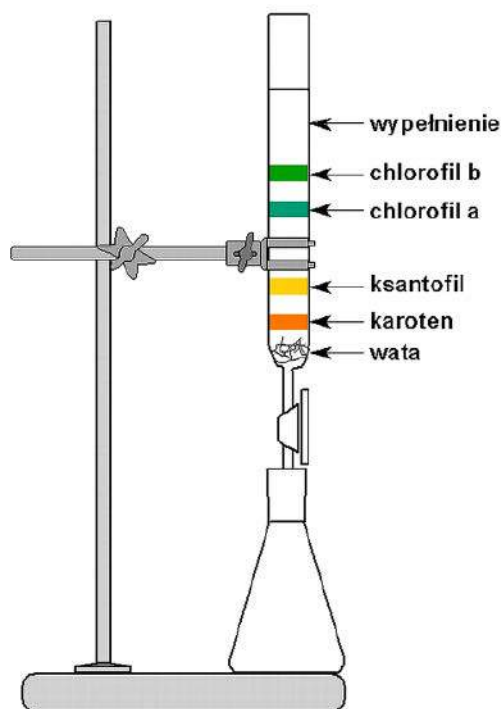
2. Rozdzielanie barwników roślinnych w kolumnie chromatograficznej (wata chroni przed zatkaniem wylotu przez wypełnienie kolumny)
