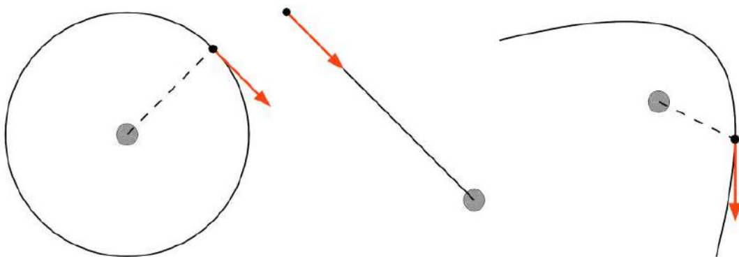
1. Linia ciągłą zaznaczono przykładowe trajektorie ciała poruszającego się w centralnym polu grawitacyjnym. Czerwona strzałka oznacza wektor prędkości, a linia przerywana – promień wodzący
